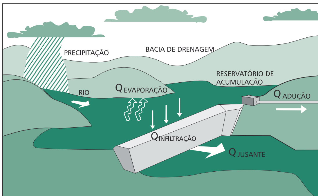
Figura 4.3 – Esquema típico de um reservatório de acumulação empregado em sistemas de abastecimento de água (adaptado de NAGHETTINI, 1999)
