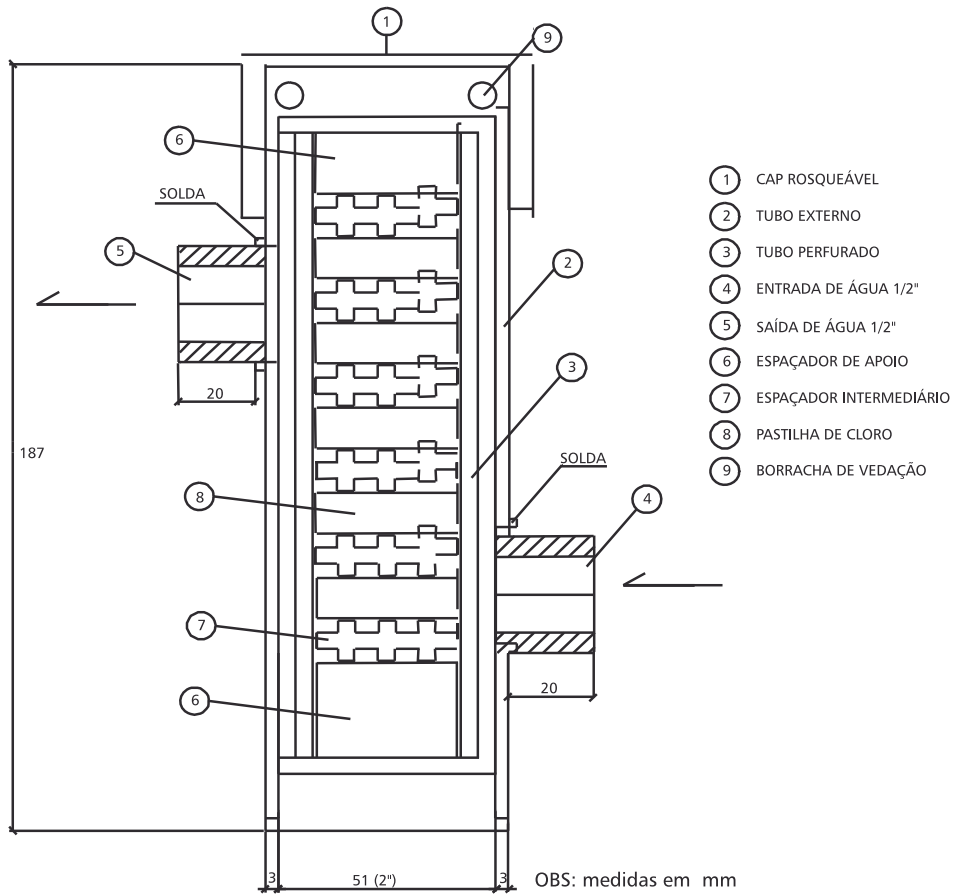
Corte A-A
